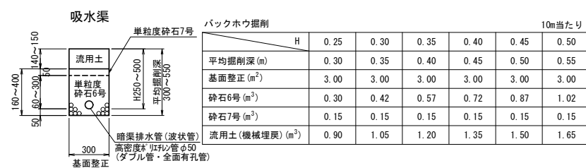
標準断面図 S=1:20
