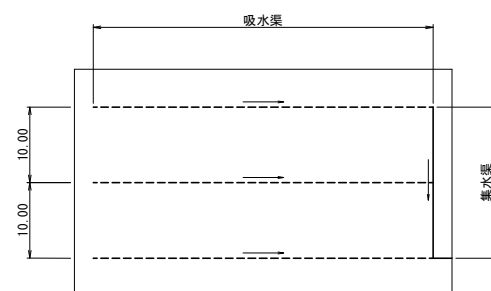
平面图 S=1:500
