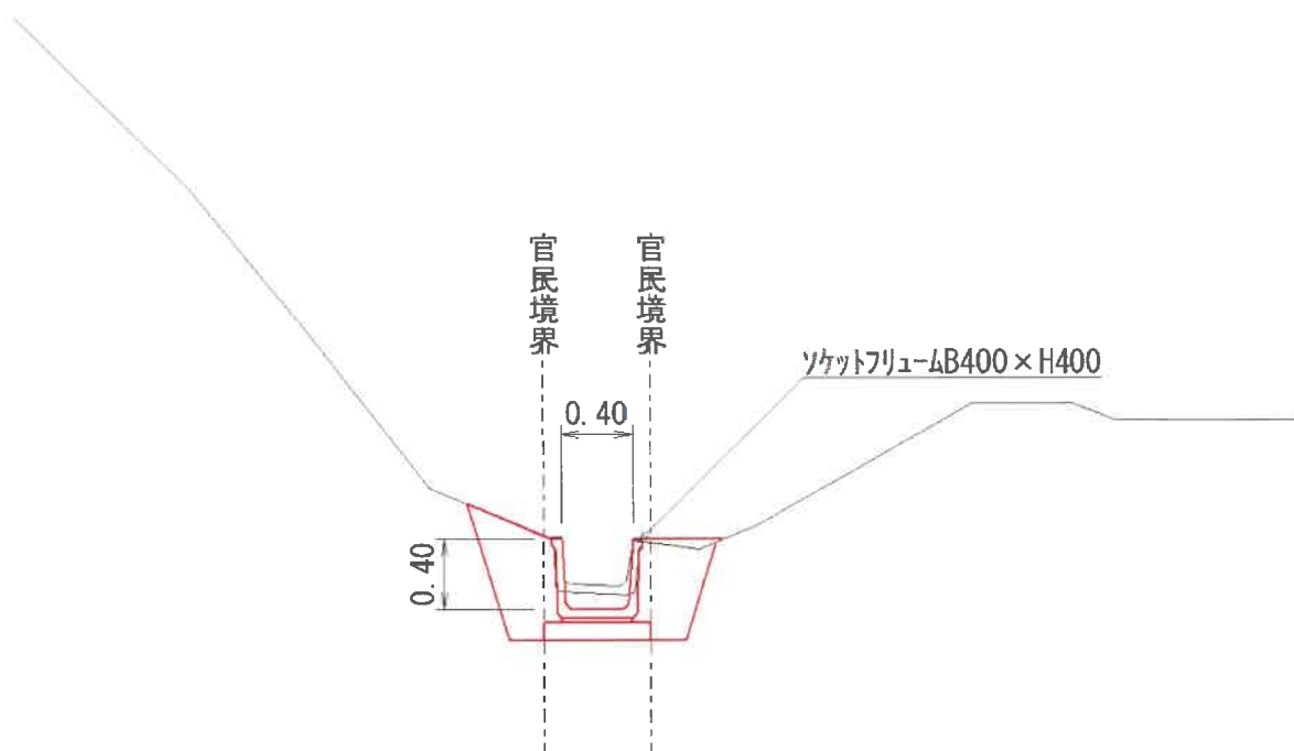
佐文 1 地区標準断面図
