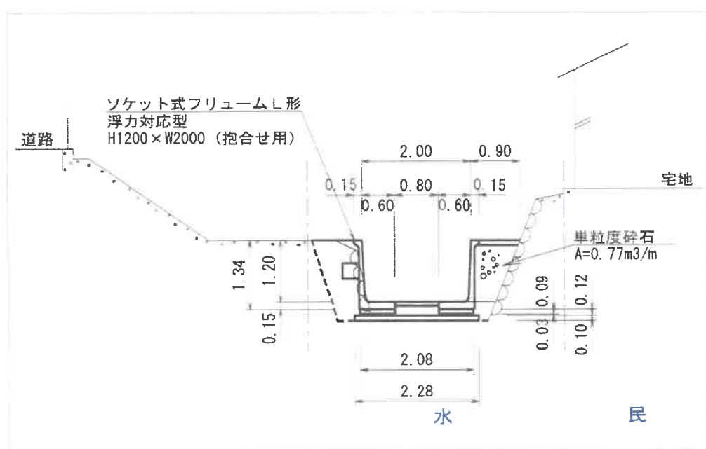
標準断面図
