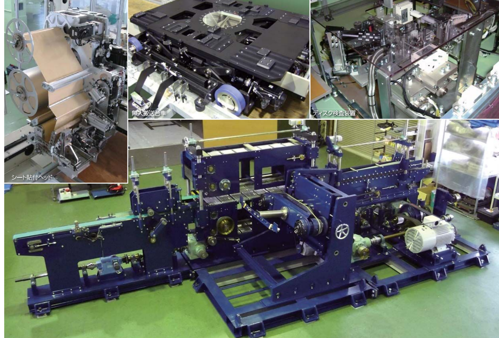
ティッシュペーパー切断機
