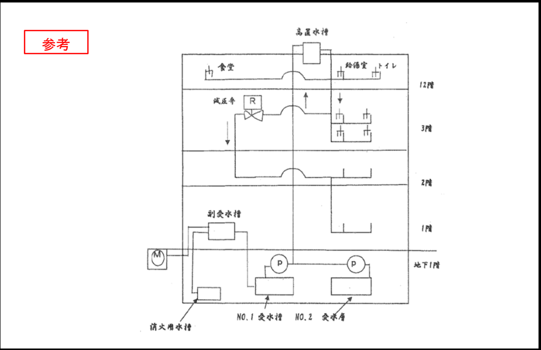
簡易専用水道系統図
