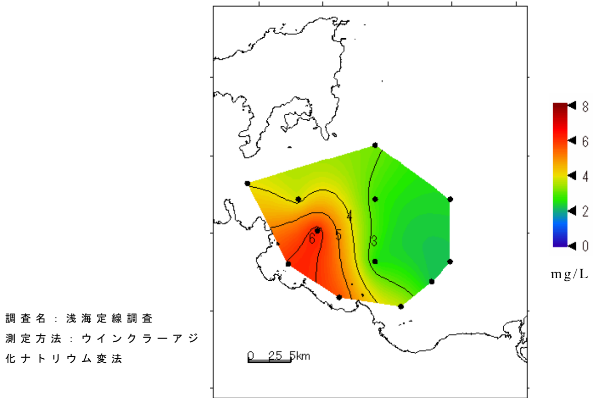
底層の溶存酸素濃度
