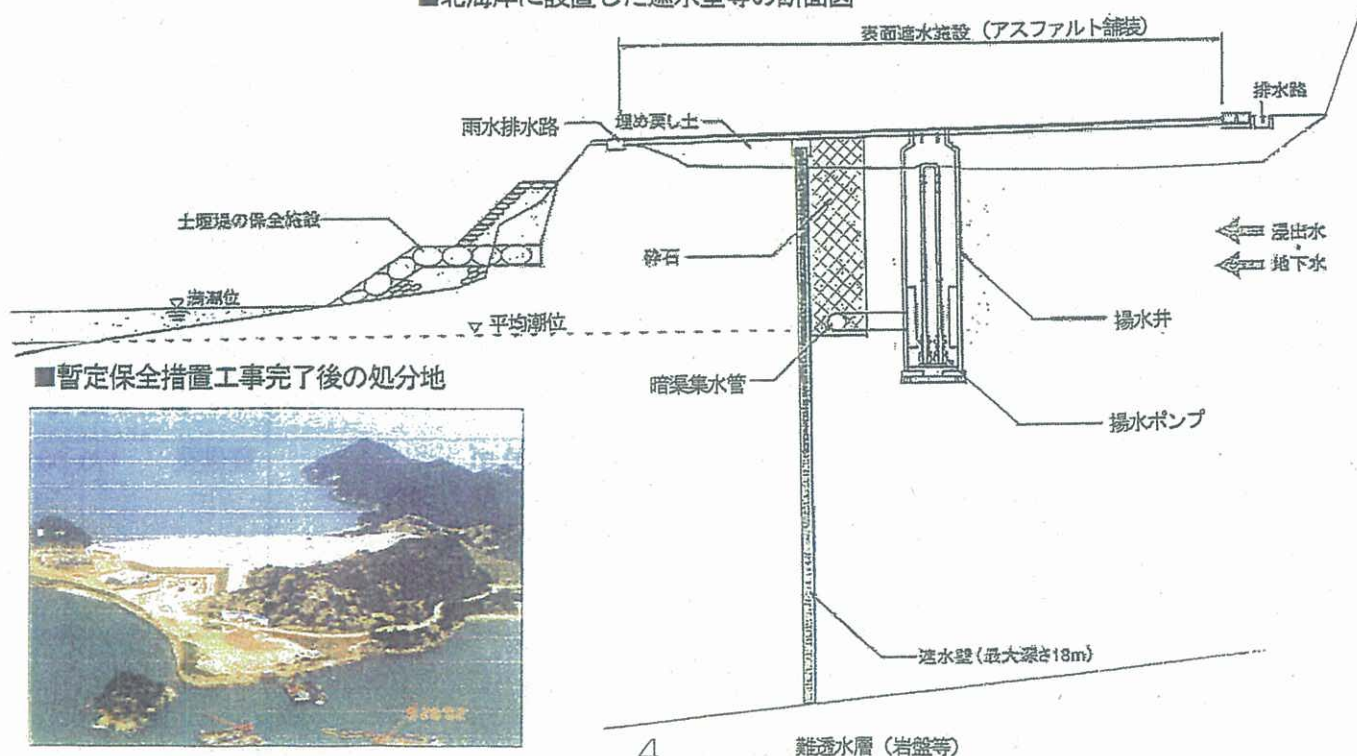
■北海岸に設置した遮水壁等の断面図
